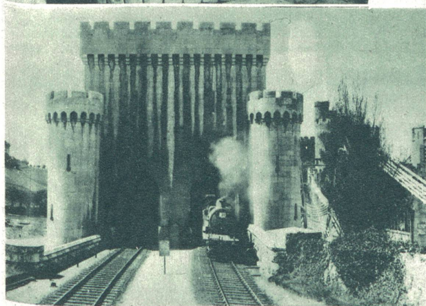
Eine Eisenbahn, die durch ein Schloß hindurchfährt. Das Schloß steht auf dem Wege nach Irland, auf der Strecke der London-Midland-Bahn, und ist eines der schönsten alten Schlösser Englands. Photo International Graphic Press.
