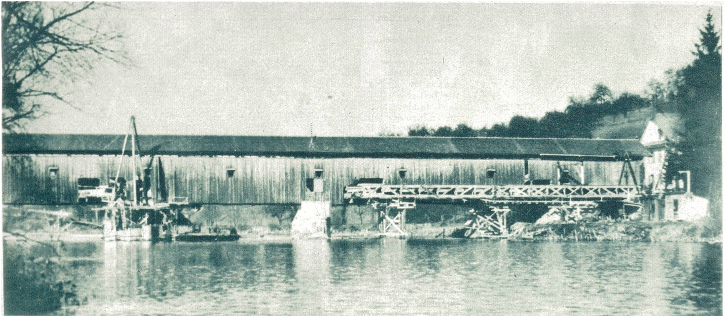
Eine historische Brücke wird niedergerissen. Die alte historische Brücke über die Reuß bei Gislikon, bekannt aus dem Sonderbundskrieg, wird niedergerissen, um einer modernen Verkehrsbrücke Platz zu machen. Unser Bild zeigt die alte Gislikoner Reußbrücke. Unmittelbar vor derselben sind die Bauarbeiten für die neue Verkehrsbrücke bereits in vollem Gange. Photopress, Zürich.
