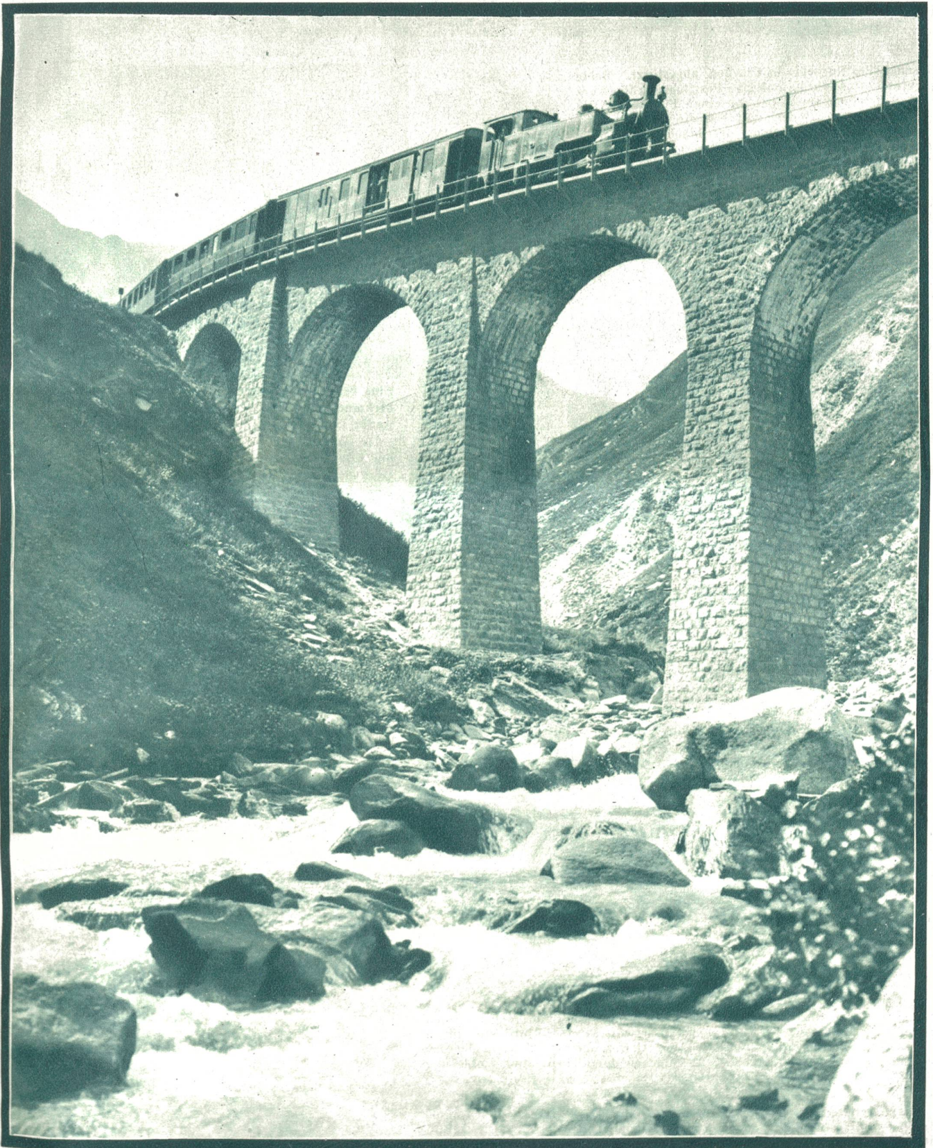
Furkareuss-Viadukt der Furka-Oberalp-Bahn hinterhalb Realp im Urserental.
