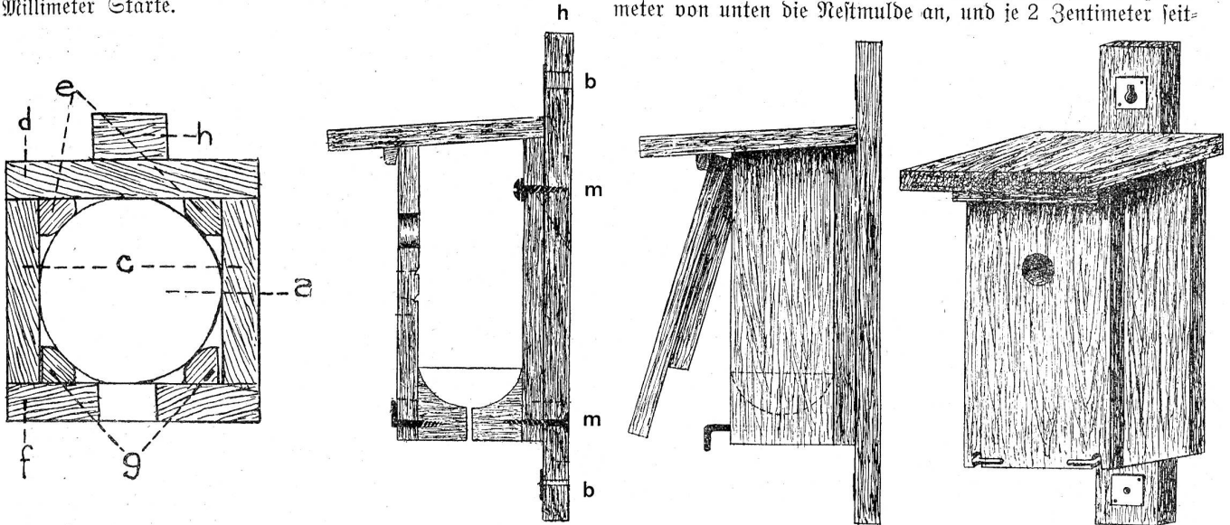
Grundriß des Ala-Nistkastens. Querschnitt durch den Ala-Nistkasten. Ala-Nistkasten. Ansicht von der Seite. Ansicht des Ala-Nistkastens.
