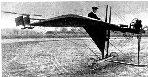
Der primitive Eindecker des Franzosen Kaufmann kam 1910 in seinem Aversieren, schon den später allgemein üblichen Formen nahe. Aber trotz seines 24 PS starken Motors hob sich der kleine Apparat nie in die Lüfte
