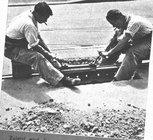
Zuletzt wird die ganze Schweißstelle, soweit sie befahren wird, mit dem Schienenhobel abgeglättet
