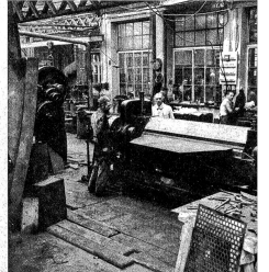
Die Plattenerschneidmaschine im Betrieb
