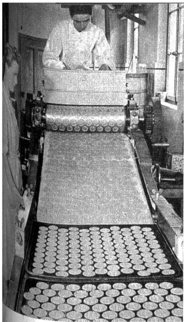
Gebäckformmaschine
