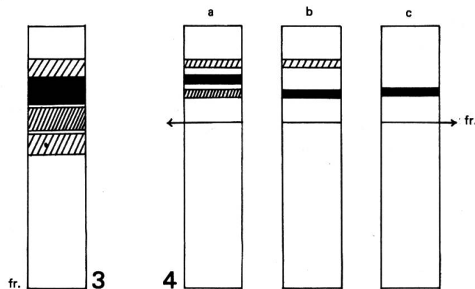
Fig. 3. — Electrophorogramme de globulines solubles. Même profil pour tous les fragments. Fig. 4. — Electrophorèse sur agarose des peroxydases. Variation selon la topographie: a = sommet; b = partie équatoriale; c = base.
