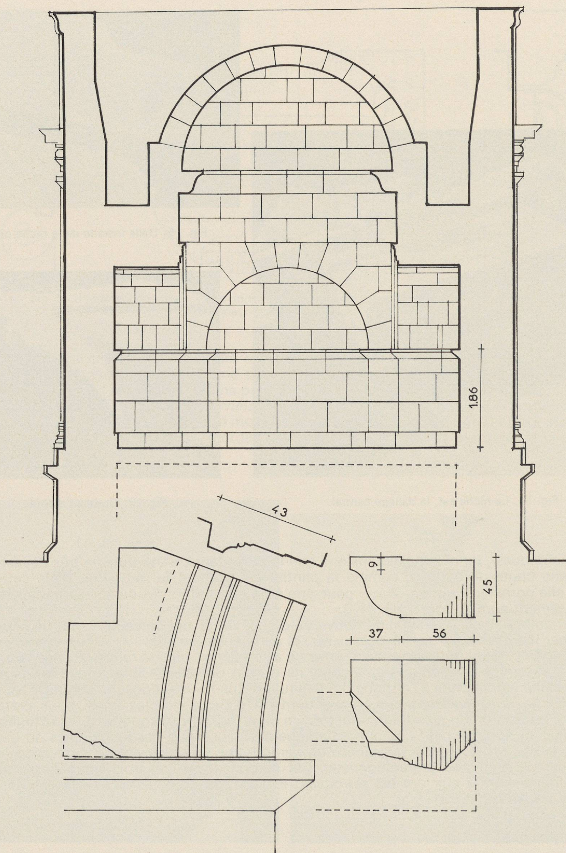
Fig. 17: Coupe transversale ouest-est restituée; en bas: arcossolium couvrant les niches; doucine d'encorbellement intérieur (corbeau).
