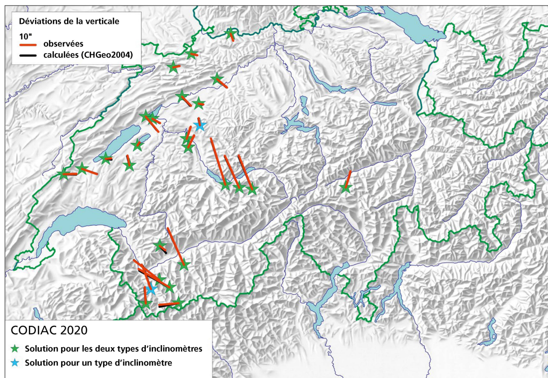
Figure 4: comparaison entre les déviations de la verticale mesurées dans le cadre de la campagne 2020 (en rouge) et celles calculées à partir du modèle de géoïde (en noir)
