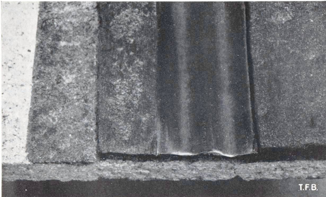
Abb. 4 Gewelltes Kupferblech in Bitumen eingebettet (sog. RISSI-Belag).
