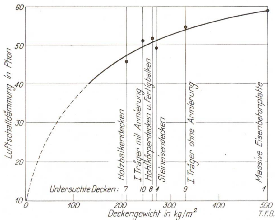
Abb. 1 Luftschallisolation in Funktion des Deckengewichts. Freigelagerte Decken von 4.20 m Spannweite
