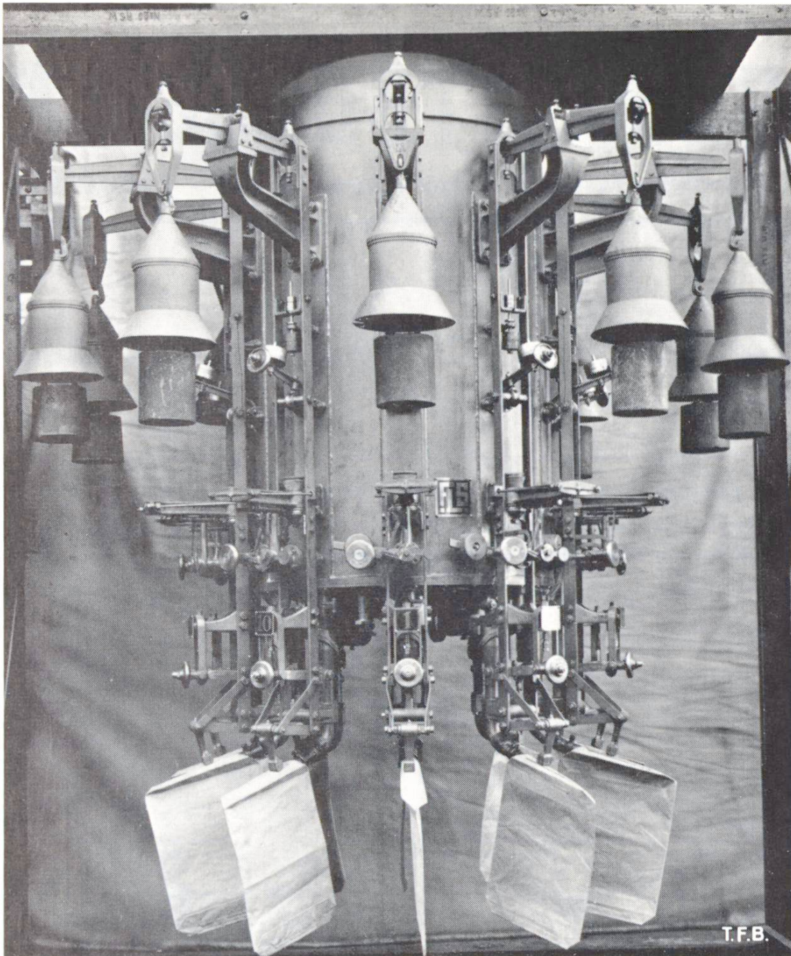
Abb. 2 Die Karussell-Packmaschine
