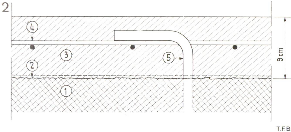
Abb. 1 Deckbelag. 1 = Konstruktionsbeton, 2 = Aufgerauhte Oberfläche, eingemörtelt, 3 = Belagsbeton BH 350, 4 = Stahldrahtnetz, 5 = Verankerung
