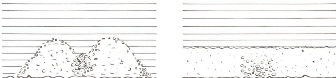
Abb. 15 Bildung von Kiesnestern bei unsachgemäßem Einbringen und Verdichten des Betons.
