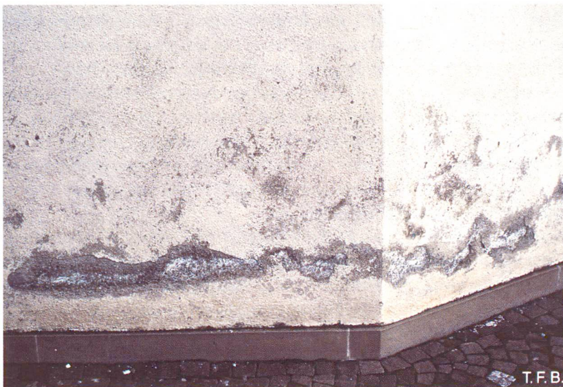
Abb. 17 Aus dem Fundament aufsteigende Feuchtigkeit mit gelösten Salzen verursacht über dem stark wasserdampfhemmenden Sockel Schäden mit Ausblühungen (Mauer aus dem 16. Jahrhundert, Alter des Verputzes: ca. 30 Jahre).
