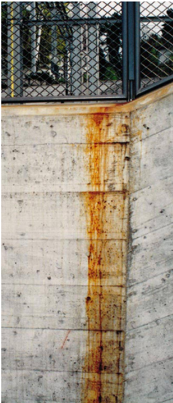
Auch Rostspuren auf Sichtbeton lassen sich entfernen (links). Mit Flechten bewachsener Sichtbeton (rechts).
