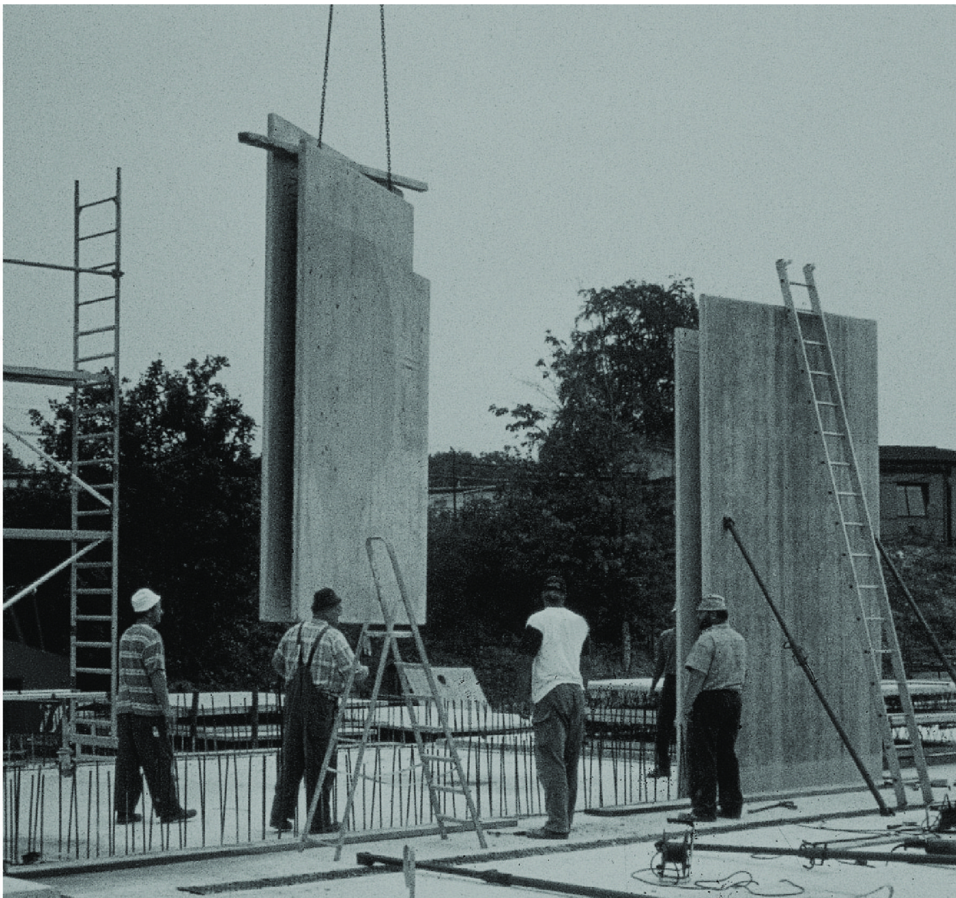
Aufstellen von Dreifachwänden.
