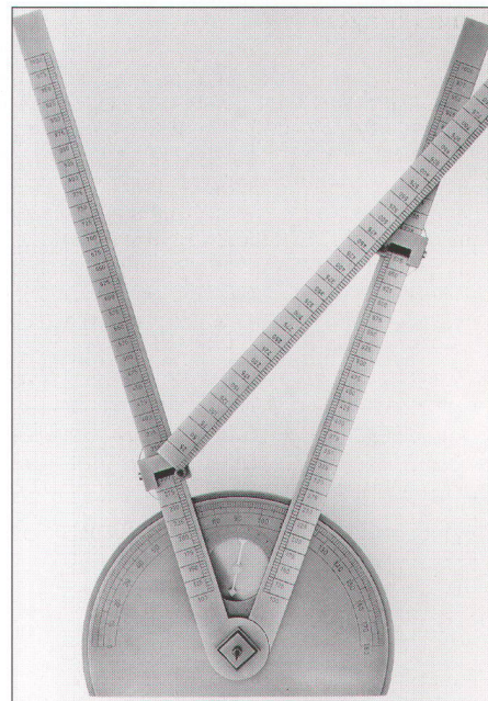
Abb. 2: Halbkreisinstrument mit zwei Alhidaden. Rekonstruktion von Erwin Minder aus Pfungen, nach Vorlagen von Leonhard Zubler, 1607 (Schweizerisches Landesmuseum, Zürich).
