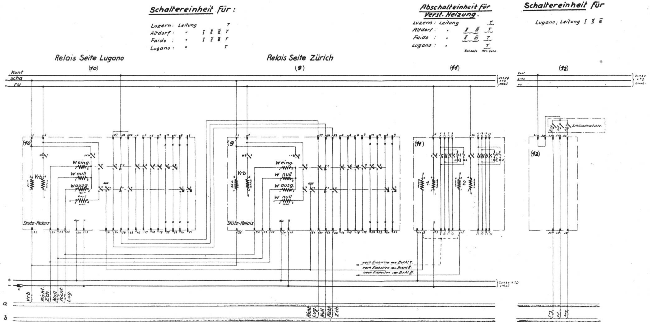
Abb. 4. Schaltung der Schaltereinheiten in den Empfangsstationen.
