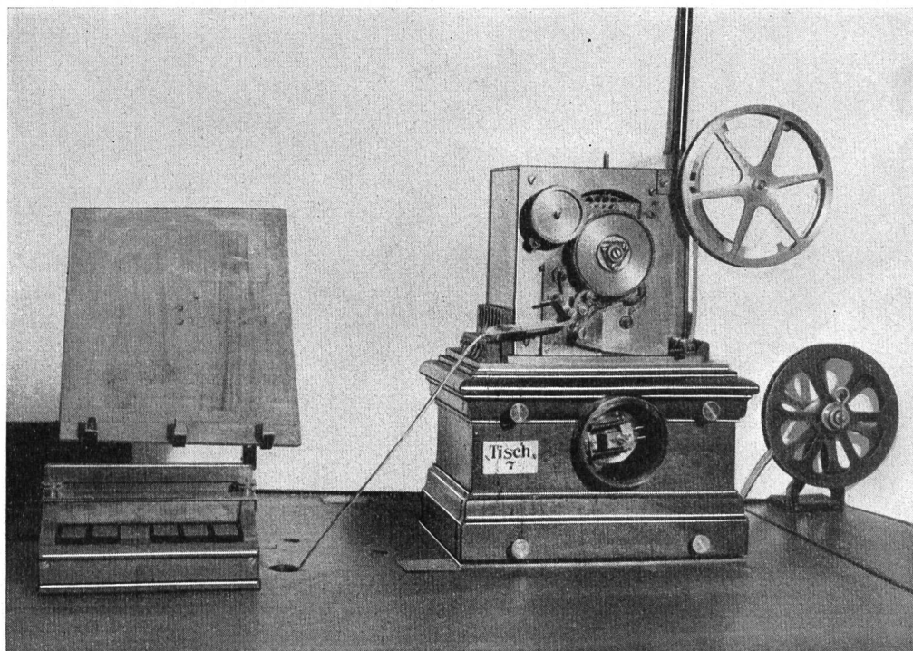
Abb. 19b. Baudot-Arbeitsplatz
