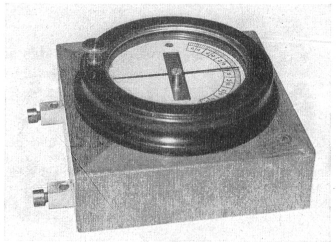
Abb. 14. Boussole
