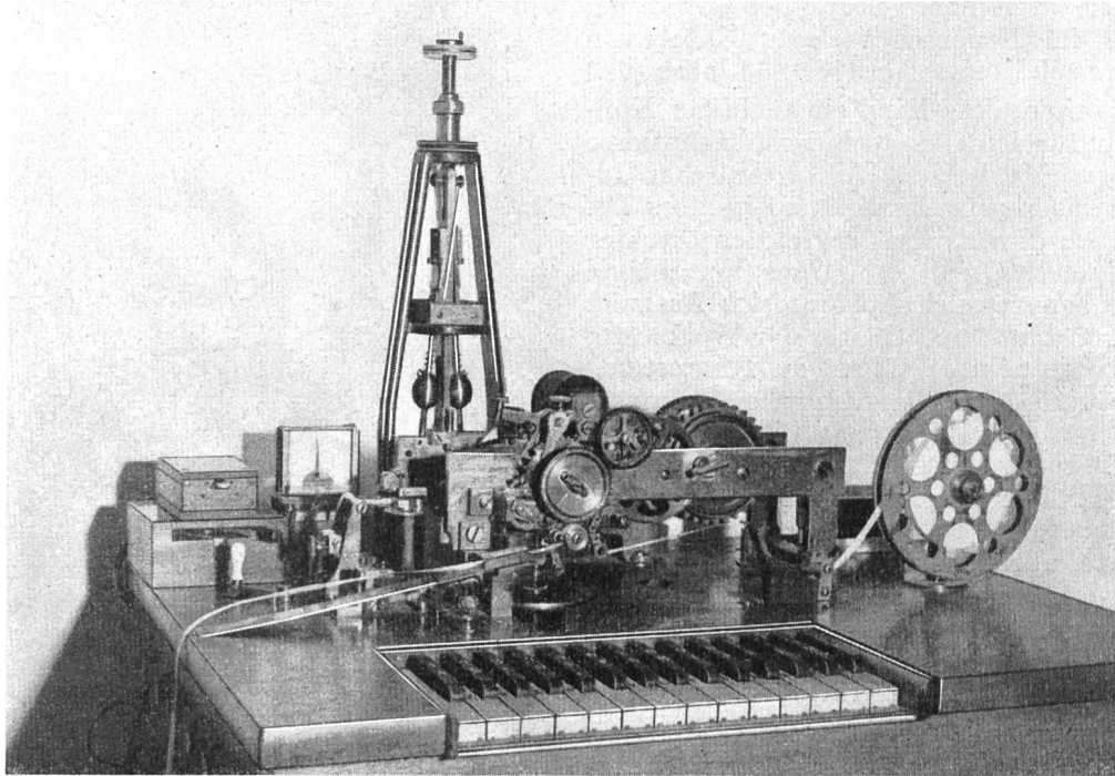
Abb. 18. Hughes-Apparat
