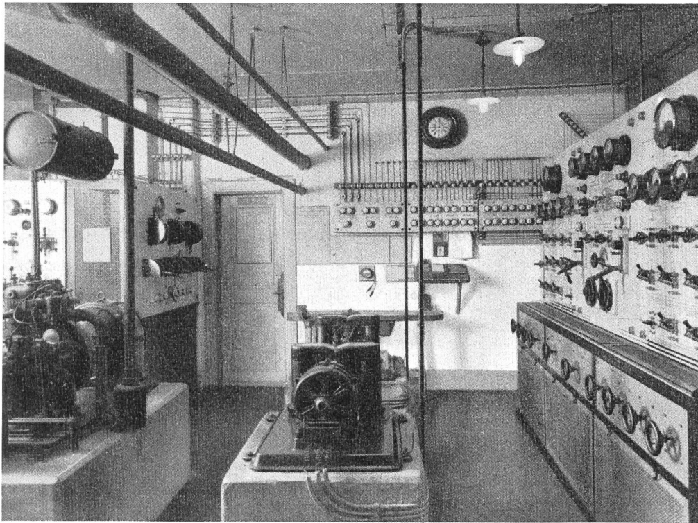
Abb. 31. Maschinenraum Zürich 1924
