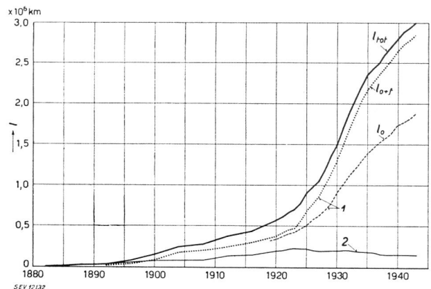
Fig. 9. Longueurs de fils du réseau téléphonique 1882...1943 l_{tot} longueur totale des fils 1 fils souterrains l_{0+f} câbles locaux et interurbains 2 fils aériens. l_0 câbles locaux
