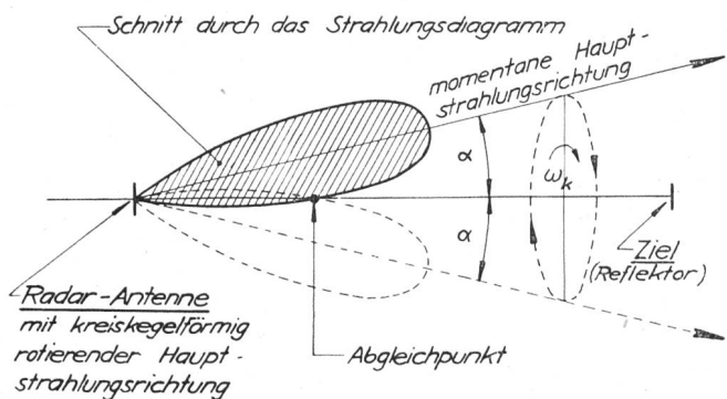
Fig. 1. Richtungsbestimmung
