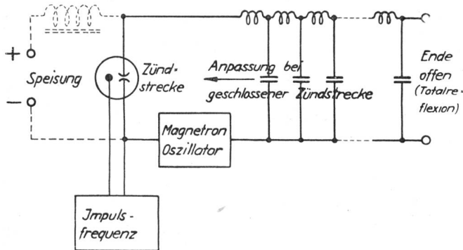
Fig. 2. Impuls-Modulationsschaltung
