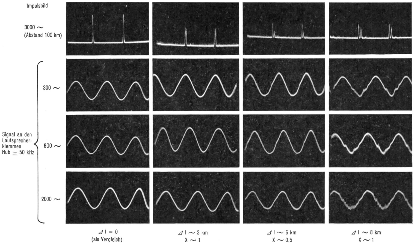
Fig. 35. Messbeispiel für Verzerrungen mit geringem Amplitudenunterschied ( x_j \rightarrow 1 ) und verschiedener Weglängendifferenz
