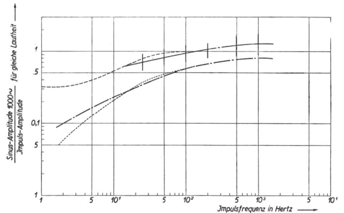
Fig. 52. Die relative Lautheit von Impulsstörungen am Ausgang des frequenzmodulierten Empfängers, verglichen mit einem Sinuston in Abhängigkeit von der Impulswiederholungsfrequenz —|—|— Gehörbeurteilung (Mittel von 4 Personen) ----- Exponentiell abklingender Knack mit einer Zeitkonstanten von 1 Millisekunde, nach Steudel - . - . - . Messung mit dem Störmessplatz nach CISPR ..... Messung mit dem Störmessplatz nach CISPR und zusätzlichem Ohrkurvensieb (Siemens)
