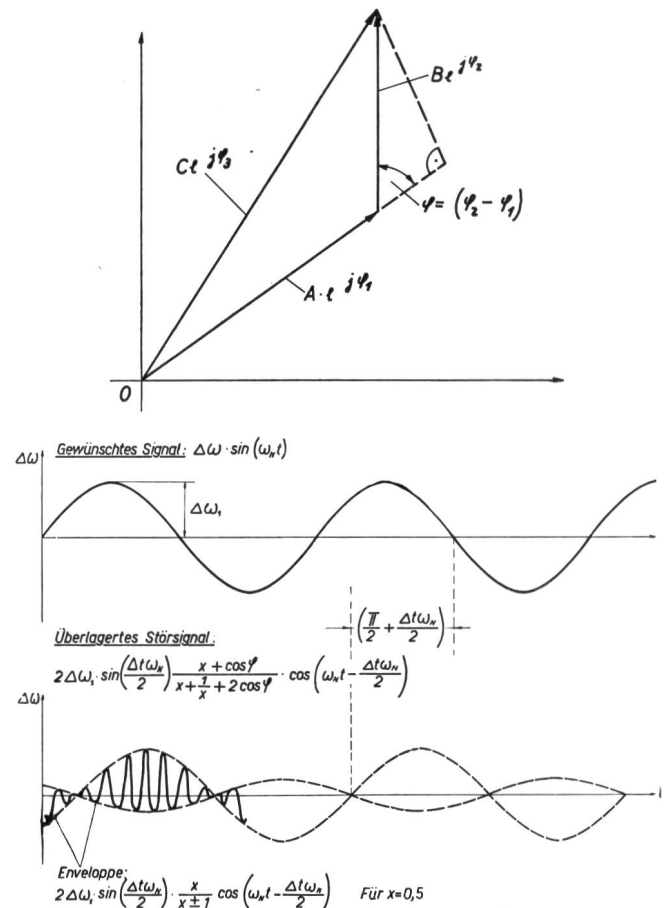
Fig. 28. Verzerrung durch Zweizege-Ausbreitung bei Modulation mit einem diskreten Ton
