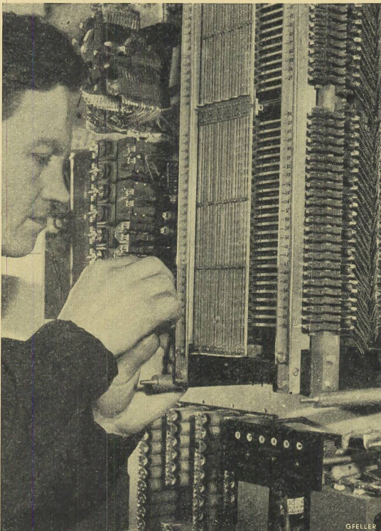
Montieren eines Kreuzwählers
