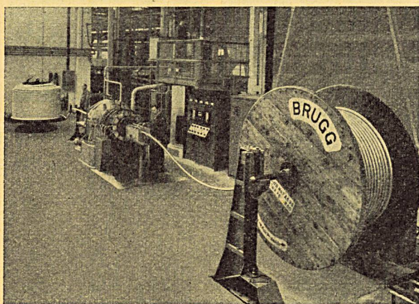
«Kontinuierliche Bleikabelpresse»
