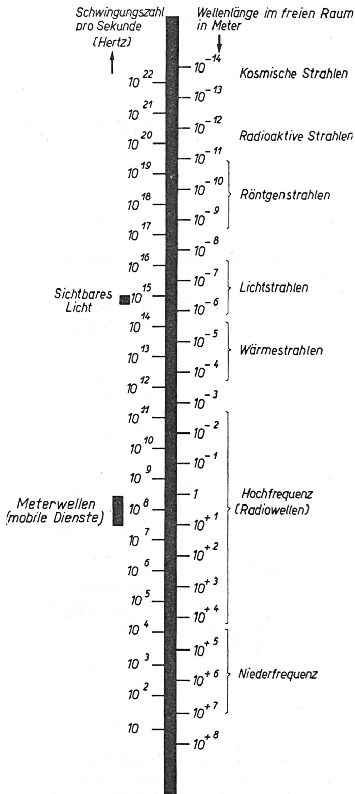
Fig. 1. Spektrum der elektromagnetischen Wellen
