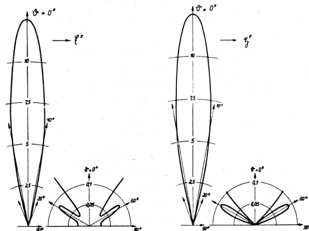
Fig. 6. Relative Intensität der gebeugten Welle in Abhängigkeit von der Strahlrichtung \vartheta für die leitende Kreisscheibe vom Durchmesser d = 3,18\lambda in der E - und H -Ebene. Fernfeld streng gerechnet (Andrejewski)
