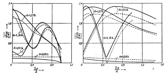
Fig. 12. Relative Schalldruckamplitude der Beugungswelle an der Oberfläche (linkes Bild) und auf der Mittelnormale (rechtes Bild) einer schallharten Kreisscheibe vom Durchmesser d = 0,08\lambda, 1,27\lambda, 1,91\lambda, 3,18\lambda
