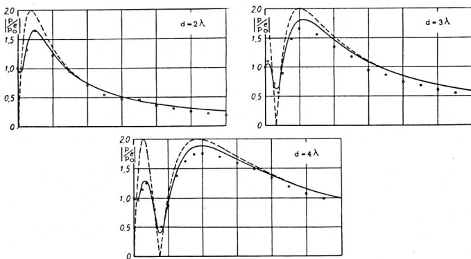
Fig. 10. Relative Schalldruckamplitude auf der Mittelnormale hinter einer kreisförmigen Öffnung vom Durchmesser d = 2\lambda, 3\lambda, 4\lambda
