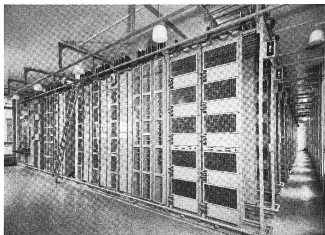
Fig. 3. Neue Zentrale Hottingen I (1953) Register, Schnurstromkreise, Prüfplatz
