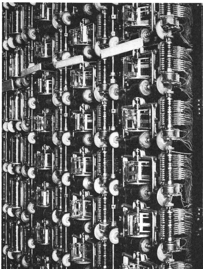
Fig. 1. Alte Zentrale Hottingen I (1917) Schnurstromkreise
