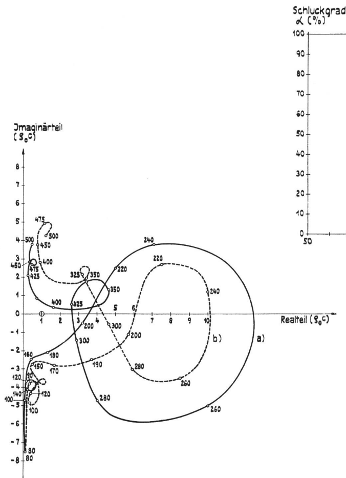
Fig. 8. Ortskurven der in Fig. 6 dargestellten Schlitzresonatoranordnung a) ungedämpft b) durch 10 mm Glaswatte schwach gedämpft
