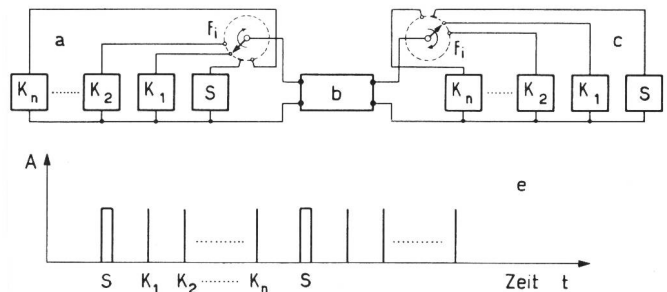
e) mit gleichem Frequenzband ausgestrahlte Pulsfolge (z.B. moduliert in der relativen Zeitlage) f_i Impulswiederholungsfrequenz, f_{K_{max}} höchste zu übertragende Kanalfrequenz, Bedingung: f_i \geq 2 \cdot (n+1) \cdot f_{K_{max}} S - Synchronisier-Kanal
