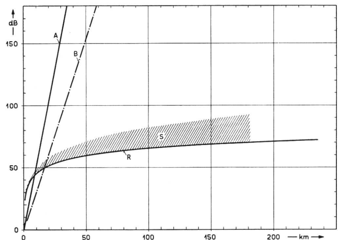
Fig. 5. Streckendämpfung mit Koaxialkabel bzw. Richtstrahlverbindung A = Koaxialkabel CCIF, \varnothing 2,6/9,4 mm, bei 5 MHz Bandbreite B = Koaxialkabel \varnothing 5/12 mm, bei 5 MHz Bandbreite R = Optimal dimensionierte Richtstrahlverbindung (Bandbreite praktisch nur durch Apparate begrenzt) F_A = 5 \text{ m}^2 , \lambda = 10 \text{ cm} S = Schwundmarge
