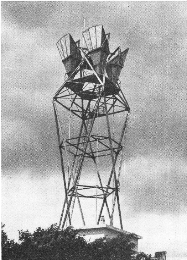
Fig. 14. Richtstrahlurm der Versuchsstation Corneilles-en-Parisis mit drehbaren Horn-Parabol-Strahlern für die Übertragung sehr breiter Frequenzbänder im Bereiche von 4000 MHz (zirka 7,5 cm Wellenlänge). Das Bild wurde uns freundlicherweise vom Service des Recherches et du Contrôle Technique des PTT, Jssy-les-Moulineux, zur Verfügung gestellt
