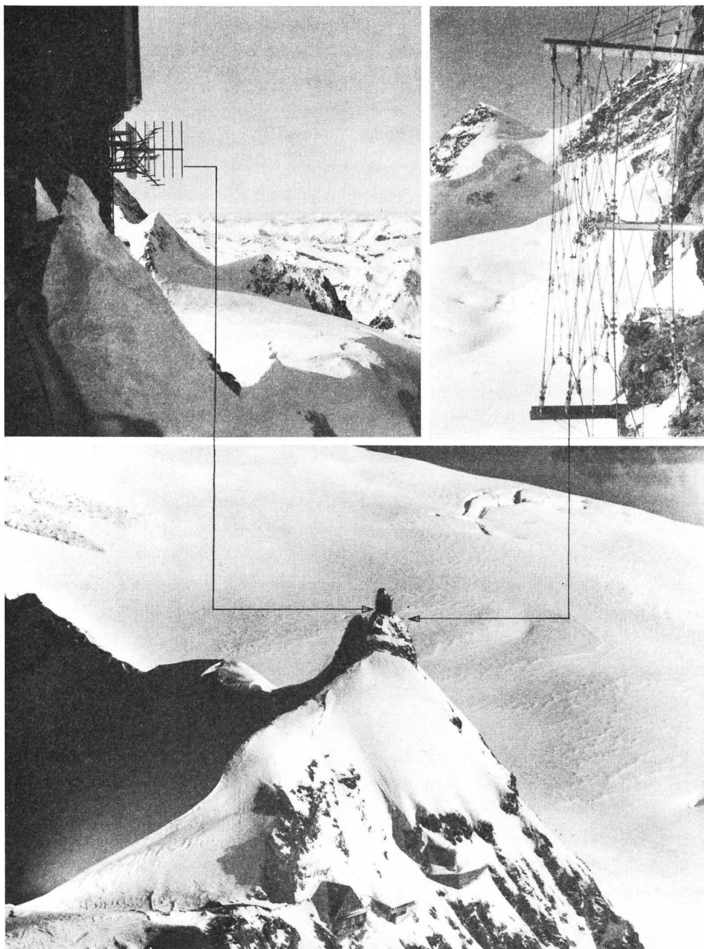
Fig. 13. Höhenstation Sphinx, Jung- frauoch, 3573 m ü. M., im Zentrum der Schweizer Alpen gelegen, ermöglichte erstmals eine kommerzielle Mehrkanal- Richtstrahlverbindung über die Alpen (Bern-Lugano, im Frühjahr 1950). Die fehlende Sicht mit der Gegenstation Monte Generoso am Alpen- südfuss bedingte hier ver- hältnismässig grosse Anten- nen in Verbindung mit der Anwendung verhältnis- mässig langer Wellen (zirka 1,5 m)
