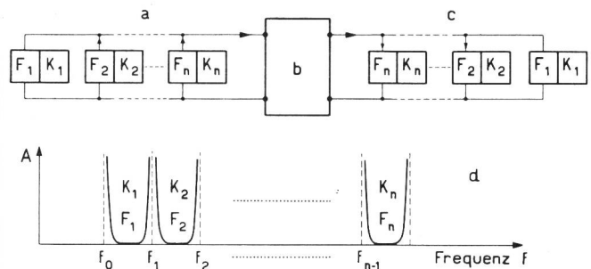
a) Sendeseite, b) Gemeinsamer Übertragungsvierpol, c) Empfangsseite d) Gleichzeitig ausgestrahltes Frequenzspektrum, F_{1..n} Kanal-Bandfilter K_{1..n} Nachrichtenkanal (in die entsprechende Frequenzlage transponiert)
