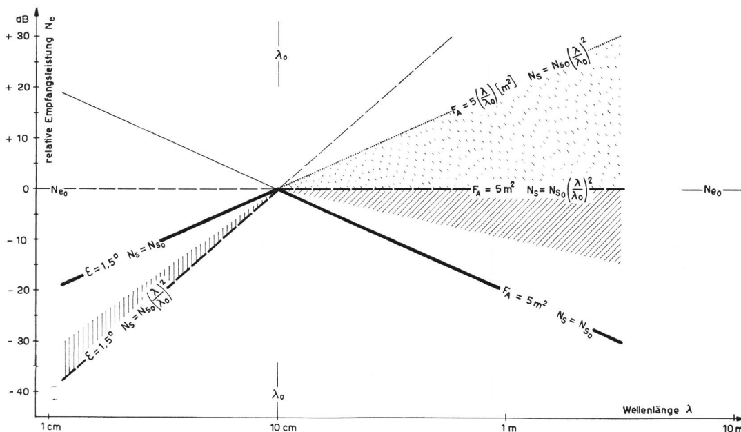
Fig. 6. Optimal verfügbare Raumwellen-Empfangsleistung bei Begrenzung der Antennengrösse und der Bündelung (für F_A = 5 \text{ m}^2 , \epsilon = 1,5^\circ ). Der schraffierte Teil entspricht etwa den heutigen Verhältnissen
