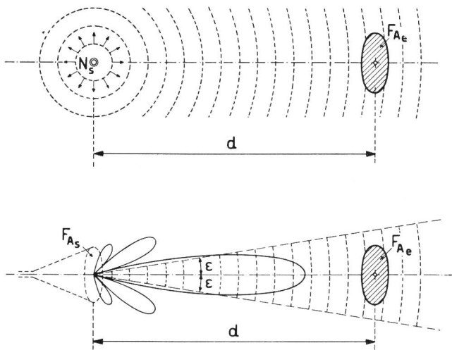
Fig. 4. Kugelstrahler und Richtstrahler F_{A_s} , F_{A_e} Absorptionsfläche der Sende- bzw. Empfangsantenne
