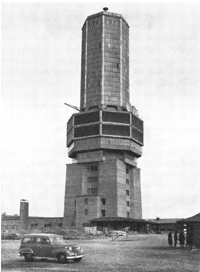
Fig. 12a. Fernmeldeturm auf dem grossen Feldberg im Taunus, 880 m ü. M., ein wichtiger Knotenpunkt des Westdeutschen Richtstrahlnetzes, gleichzeitig Stützpunkt für bewegliche Ultrakurzwellendienste (Landstrassenfunk) und Versuchszentrum. Turmhöhe 68 m. Der obere Teil ist aus Holz und enthält die umfangreicheren UKW-Antennen Das Bild wurde uns freundlicherweise vom Fernmelde-technischen Zentralamt in Darmstadt zur Verfügung gestellt
