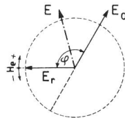
Fig. 11. Bodenreflexion und Antennenhöhe
