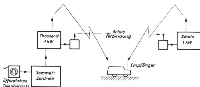
Fig. 1. Prinzipschema der Autorufanlage. Schéma de principe de l'installation d'appel des automobiles: öffentl. Telephonnetz = réseau téléphonique public Sammelzentrale = central collecteur Relaisverbindung = jonction-relais Empfänger = récepteur
