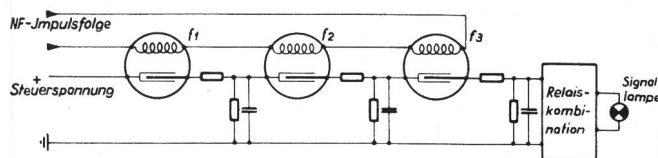
Fig. 4. Prinzipschema einer Selektiv-Automatik Schéma de principe d'un dispositif automatique de sélection NF-Impulsfolge = série d'impulsions BF Steuerspannung = tension de commande Relais-Kombination = combinaison de relais Signallampe = lampe-signal
