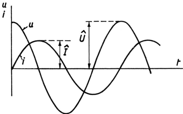
Fig. 2. Verlauf von Spannung u und Strom i beim verlustfreien Schwingungskreis (harmonische Schwingungen)
