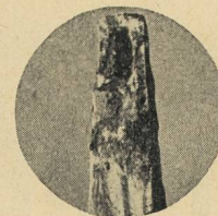
Kupferspitze nach ca. 1400 Normal- lötungen
