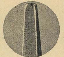
Kupferspitze nach ca. 25 000 Lötungen mit ELSOLD
