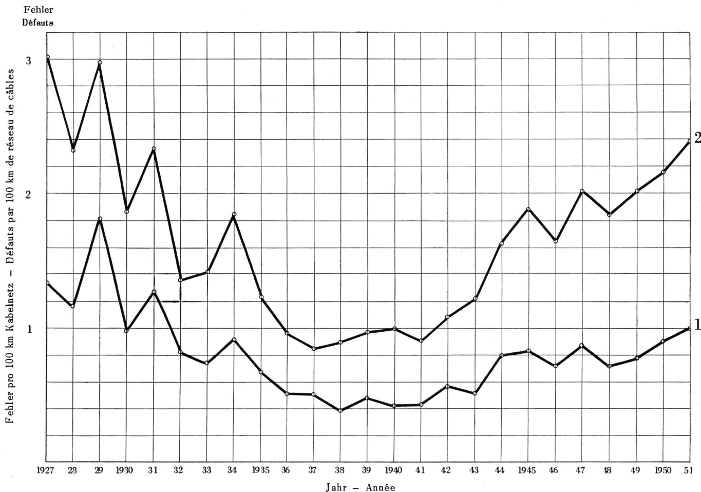
Fig. 8. Verhältnis der Zahl der Kabelfehler zu 100 km Kabelnetz - Nombre relatif des défauts de câbles par 100 km de réseau
