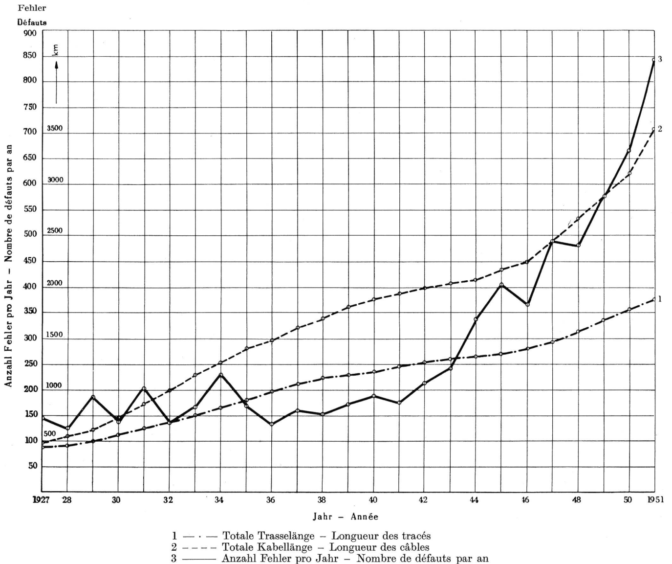
Fig. 2. Zahl der Fehlermeldungen pro Jahr - Nombre des avis de défaut par an
