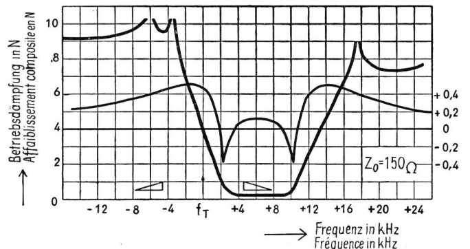
Fig. 19. Betriebsdämpfungs-Charakteristik eines 2. Modulationsfilters Caractéristique de l'affaiblissement composite d'un filtre de 2 e modulation Z_0 = Nennwert des Wellenwiderstandes Valeur nominale de l'impédance caractéristique f_T = Trägerfrequenz Fréquence porteuse
