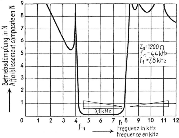
Fig. 18. Betriebsdämpfungs-Charakteristik eines 1. Modulationsfilters Caractéristique de l'affaiblissement composite d'un filtre de 1 re modulation Z_0 = Nennwert des Wellenwiderstandes Valeur nominale de l'impédance caractéristique f_1, f_{-1} = Theoretische Grenzfrequenzen Fréquences limites théoriques
