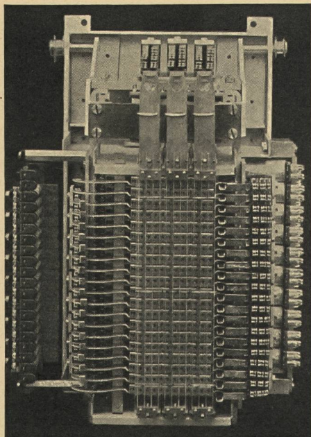
Kreuzwähler, Typ 53
