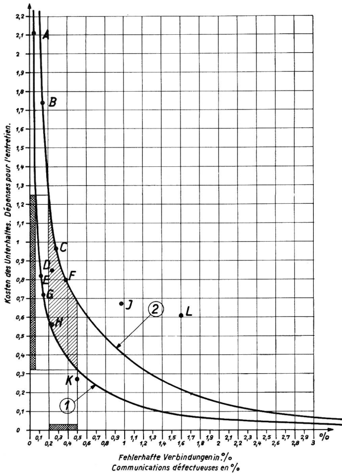
Fig. 1. Centraux automatiques. Courbe de variation de la qualité du service téléphonique local par rapport aux dépenses pour l'entretien. 1 = Centraux de construction récente. 2 = Centraux ayant 15 à 20 ans de service.
