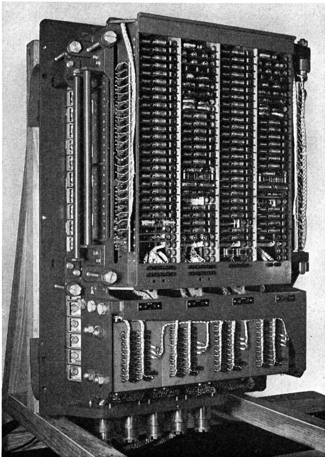
Fig. 1. Gesamtansicht des voll-elektronischen Telephonauten mit 20 Teilnehmeranschlüssen Autocommutateur téléphonique à 20 lignes entièrement électronique
