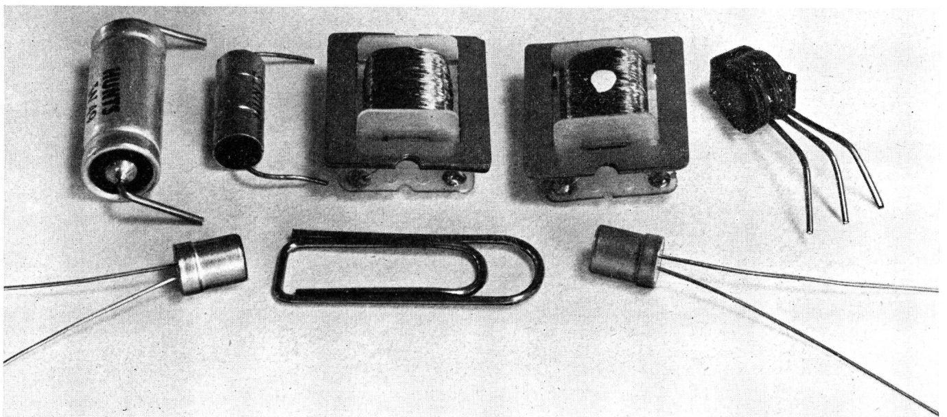
Fig. 2. Die wichtigsten Bauelemente des elektronischen Telephonauten Les principaux éléments de l'autocommutateur téléphonique électronique
