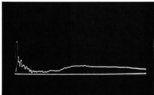
Fig. 11. Einfluss des Erdungswiderstandes eines Vorableiters in 465 m Abstand vor einer Kabelstange auf den in das Kabel übertretenden Strom.
