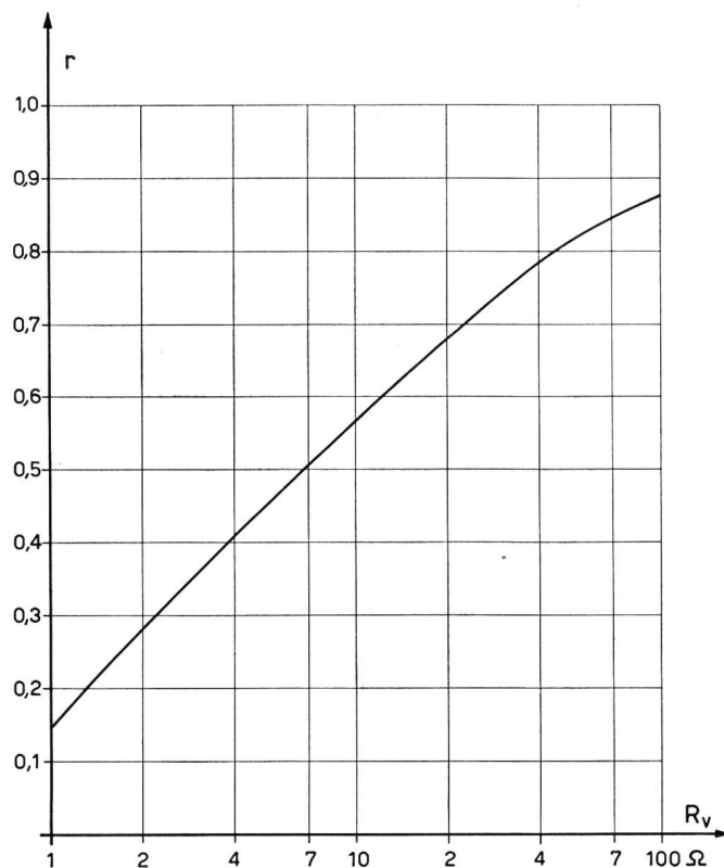
Fig. 13. Reduktion der Spannungsbeanspruchung eines Kabels durch einen Vorableiter in 465 m Abstand von der Kabelstange (Auswertung der Oszillogramme Fig. 11)
