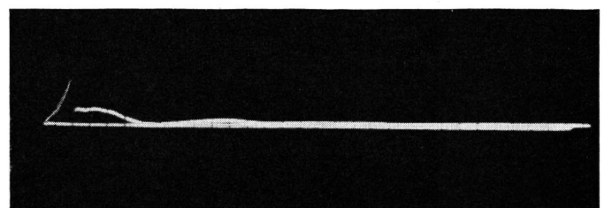
Fig. 9 a oben. Durch gewöhnlichen Edelgasableiter begrenzter Spannungsschoss 1/50 von 3 kV Scheitelwert
