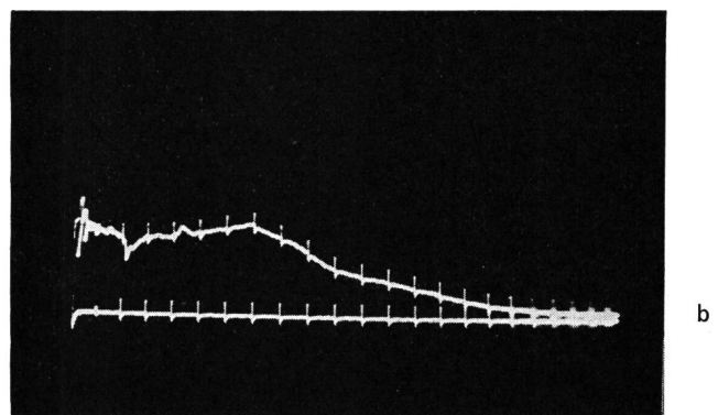
Fig. 12. Influence de la résistance de terre d'un parafoudre avancé. Avec une résistance de 20\ \Omega et à une distance de 80 m du point de transition le facteur de réduction est de 0,9 environ, c'est-à-dire insignifiant. Le point de transition se trouvait à proximité immédiate d'un central dont la résistance de terre (y compris la ligne et les résistances de mesure) valait 1,9\ \Omega . Avec un câble plus long le facteur de réduction serait un peu meilleur.
