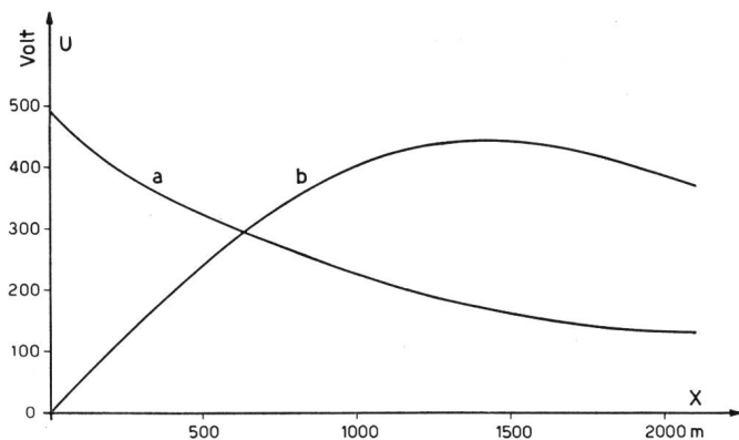
Fig. 5. Grösse der Amplitude der Spannung zwischen Bündel und Mantel in Abhängigkeit von der Entfernung x vom Einschlagpunkt. (Stromstoss und Kabeldaten siehe Fig. 4, Stromeintritt fern von den Kabelenden)
