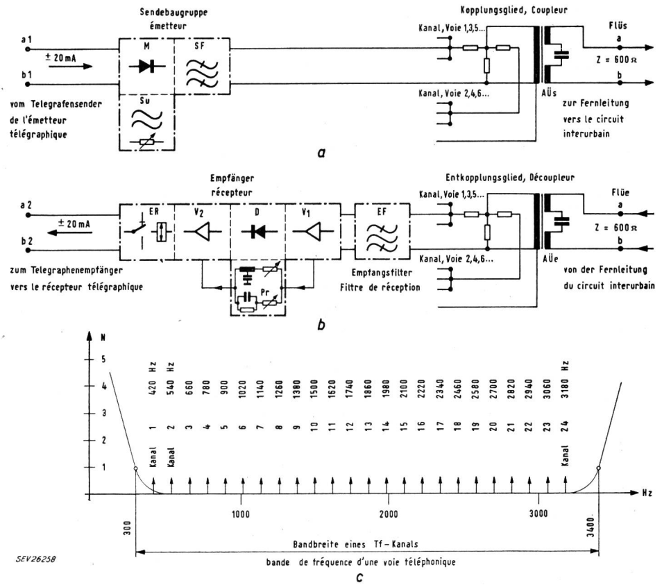
Fig. 10. Spectre de fréquences d'une voie de télégraphie harmonique et schéma de principe de l'émetteur et du récepteur d'une extrémité de voie a Schéma de principe de l'émetteur d'une voie de télégraphie harmonique; b schéma de principe du récepteur d'une voie de télégraphie harmonique; c répartition des 24 voies d'un système de télégraphie harmonique dans la bande de fréquence d'une voie téléphonique
