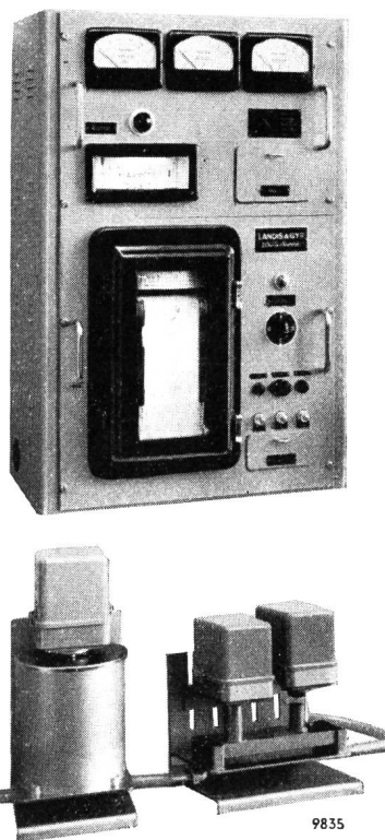
Fig. 3. Anlage zur Überwachung des Abwassers von Reaktoren, industriellen Betrieben und Laboratorien, die mit radioaktiven Isotopen arbeiten
