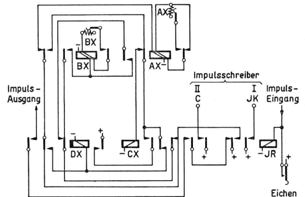
Fig. 7. Schaltbild des Stromkreises zur Kontrolle der durch den zu prüfenden Stromkreis selbst erzeugten Vorwärts- und Rücksignale auf minimale und maximale Dauer von 80...120 ms
