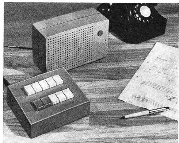
Fig. 5. Vivavox-Hauptstation: Das Lautsprecher-Mikrophon im Kunststoffgehäuse kann wahlweise auf dem Tisch aufgestellt oder an der Wand befestigt werden. Die Tastatur enthält die grüne Sprechstaste, die rote Ausschaltstaste und die weissen Teilnehmertasten
