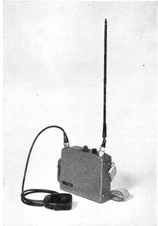
Fig. 4. SE-18-Funktelefon. Oben Anschluss für Bedienungsgerät, Kanalwähler, Squelch-Schalter, Antennenanschluss. Links vorne Monophon mit Sprechstaste, Rufstaste und Ein-Aus-Schalter
