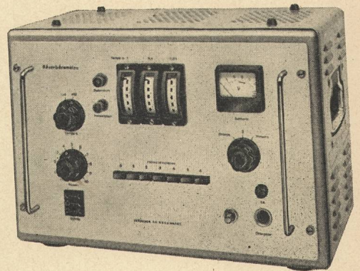
Réverbéromètre, Type B-710 Nachhallzeit-Messer, Typ B-710
