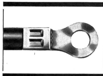
aufgepresst mit AMP-Präzisionswerkzeug
