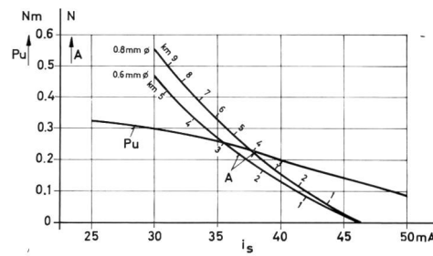
Fig. 20 Verstärkungsgrad p_u des Mikrofonverstärkers und Restdämpfungen A von Teilnehmerleitungen bei f = 800 Hz in Funktion des Schlaufenstromes i_s Gain p_u de l'amplificateur microphonique et équivalents A de lignes d'abonnés à f = 800 Hz en fonction du courant de boucle i_s
