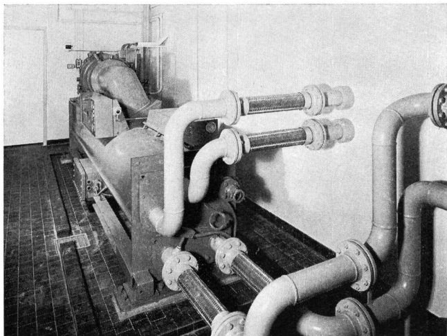
Fig. 10 Turbokältemaschine
